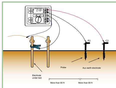
Figura 8: conexiones para la medida selectiva de electrodos de puesta a tierra
