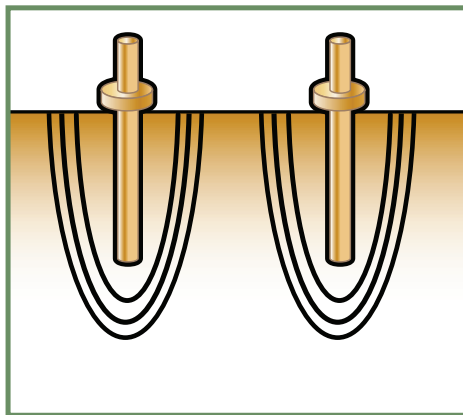
Figura 2: los electrodos de conexión a tierra tienen "áreas de influencia" a su alrededor.
