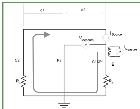
Figura 5. Circuito eléctrico de la medida
