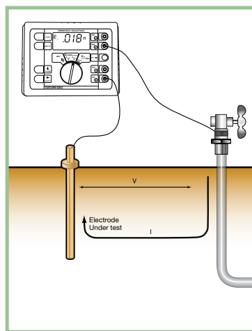
Figura 12: Configuración de la prueba en el método bipolar
