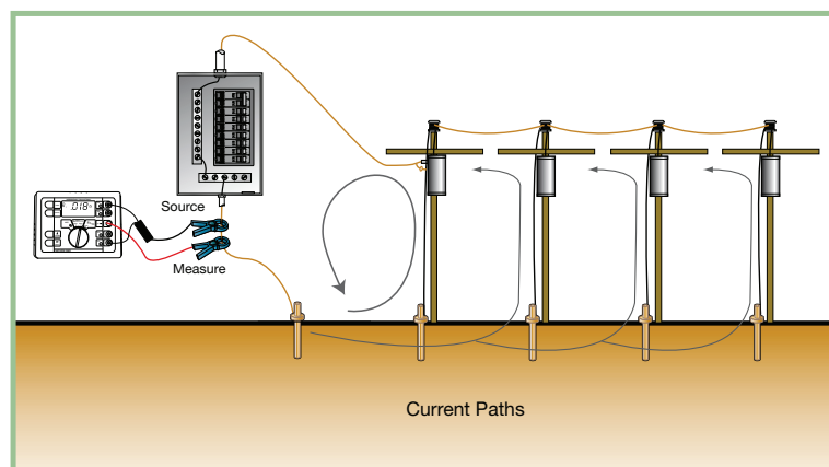
Figura 11: rutas de corriente de comprobación en el método sin picas
