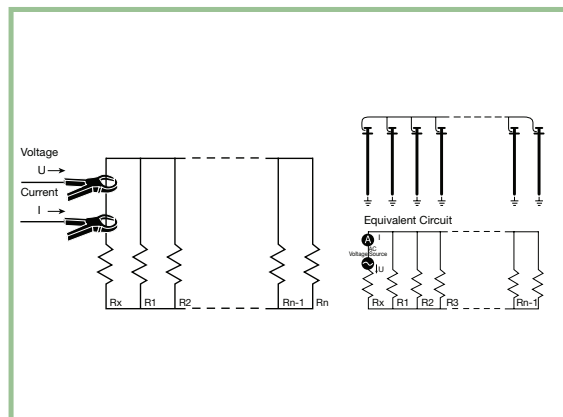
Figura 10: conexiones para la medida sin picas de la impedancia del electrodo
