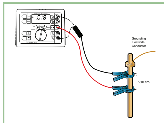
Figura 9: conexión del equipo Saturn GEO X para una medida sin picas
