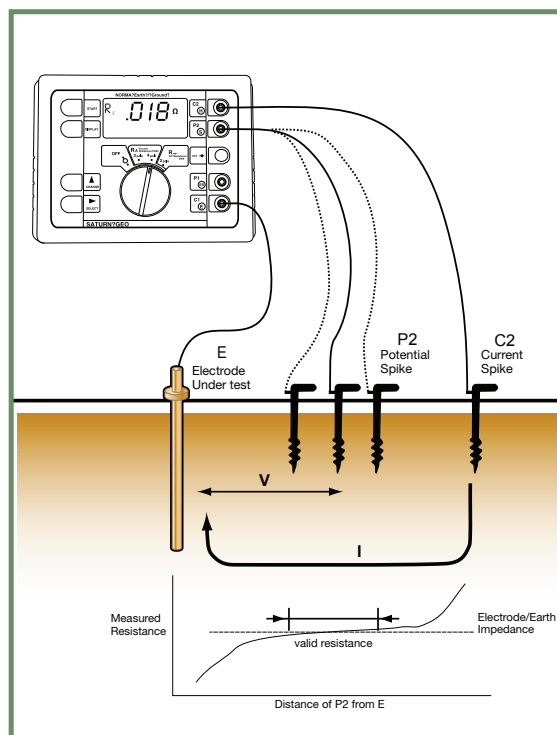
Figura 4. Esquema de conexión del telurómetro
