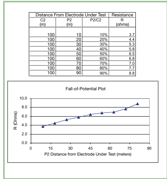
Figura 7: la impedancia de la tierra se puede obtener de la curva mediante la técnica de la pendiente de Tagg
